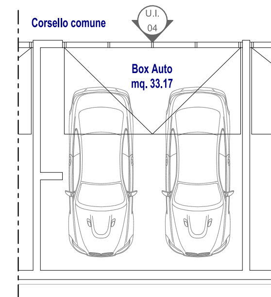
PIANO INTERRATO scala 1:100
