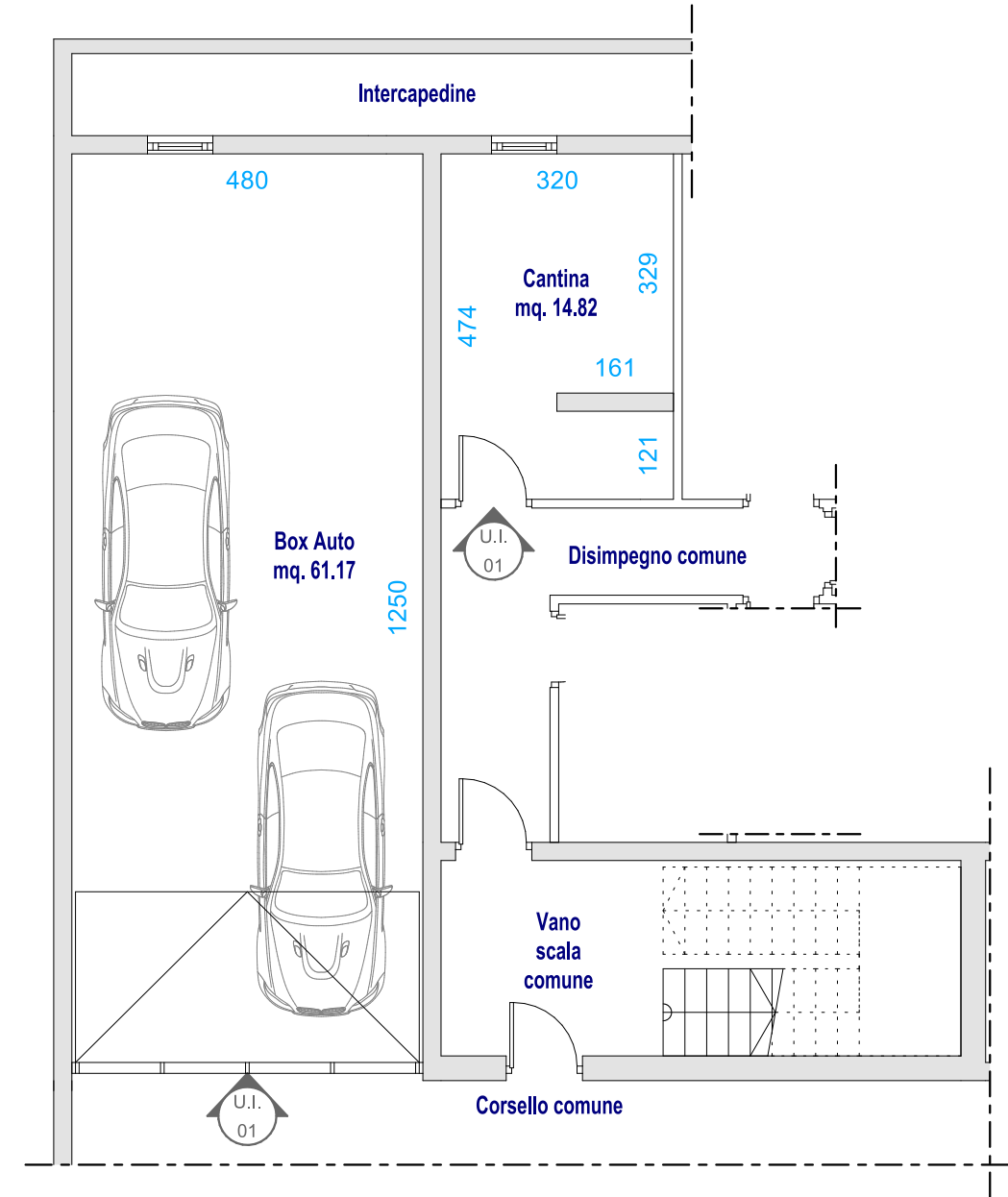
PIANO INTERRATO scala 1:100
